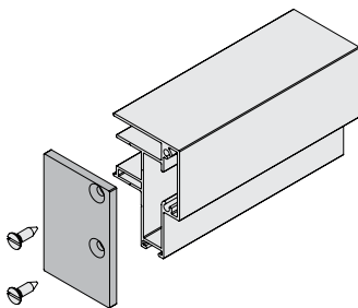
Під бокову заглушку без стійок Системи SW, SHW
