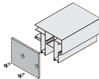
Під бокову заглушку без стійок Системи DW, DHW
