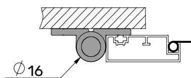
Петля 231.100 для монтажу на проєм
