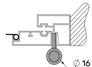
Петля 231.200 для монтажу в проєм або коробку
