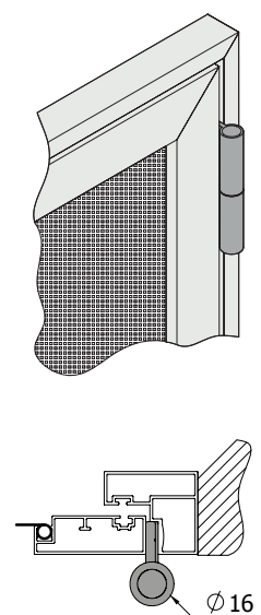
Петля 231.200
