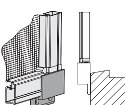
Кріплення кутове пластикове 210.200
