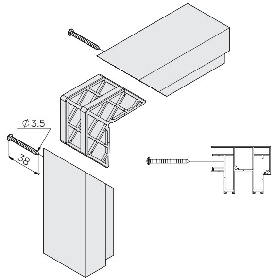
Профіль 240.200
