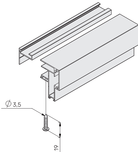
Профіль 240.100/242.000
