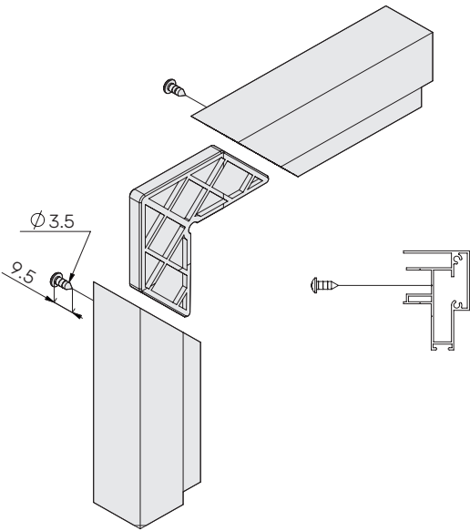
Профіль 240.100
