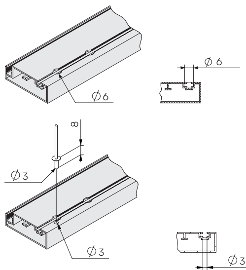
Послідовність отворів
