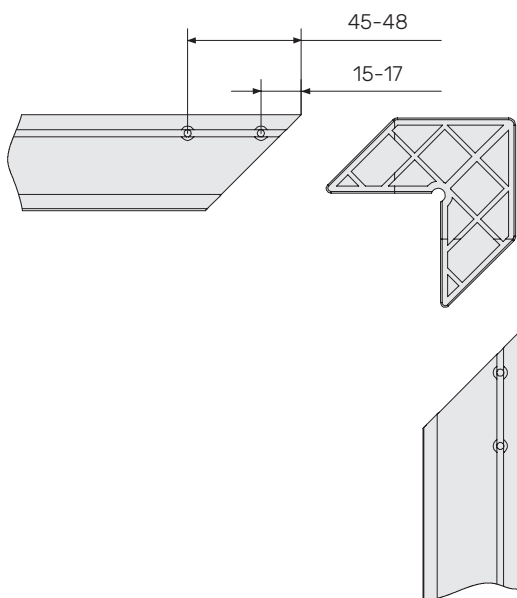
Розташування отворів на профілі для кріплення кутника
