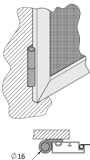
Петля 231.100S з фланцями на одну сторону
