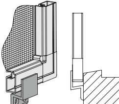
Кріплення пластикове 210.100
