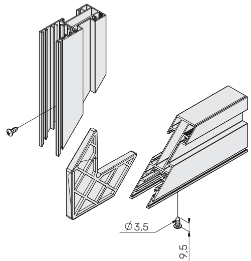
Профіль 201.158/201.058
