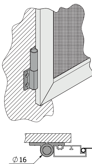
Петля 231.100 з фланцями на дві сторони
